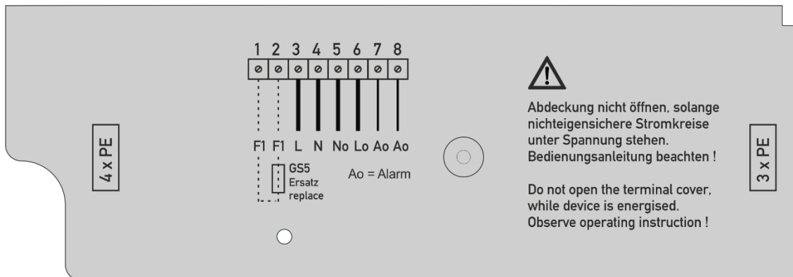
Abb. 3: Klemmenabdeckung mit Anschlussbild Baureihe 1076
